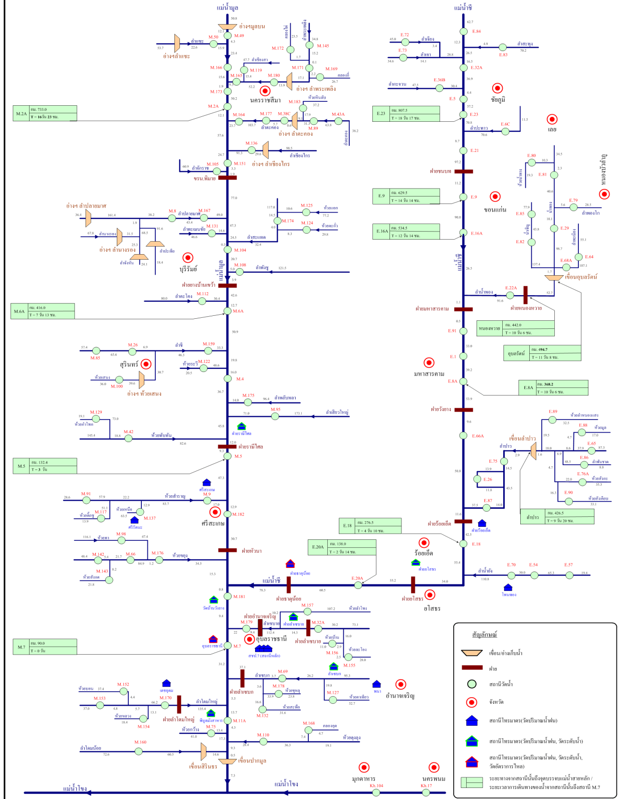
แผนภาพที่ 11 ผังเส้นทางการเดินทางของน้ำในระบบลุ่มน้ำมูลและลุ่มน้ำชี ที่มา : ศูนย์ประมวลผลวิเคราะห์สถานการณ์น้ำ กรมชลประทาน (2554)
