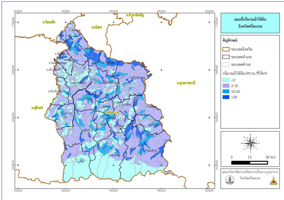
แผนภาพที่ ๑๔ แผนที่แสดงปริมาณน้ำใต้ดินของจังหวัดศรีสะเกษ
