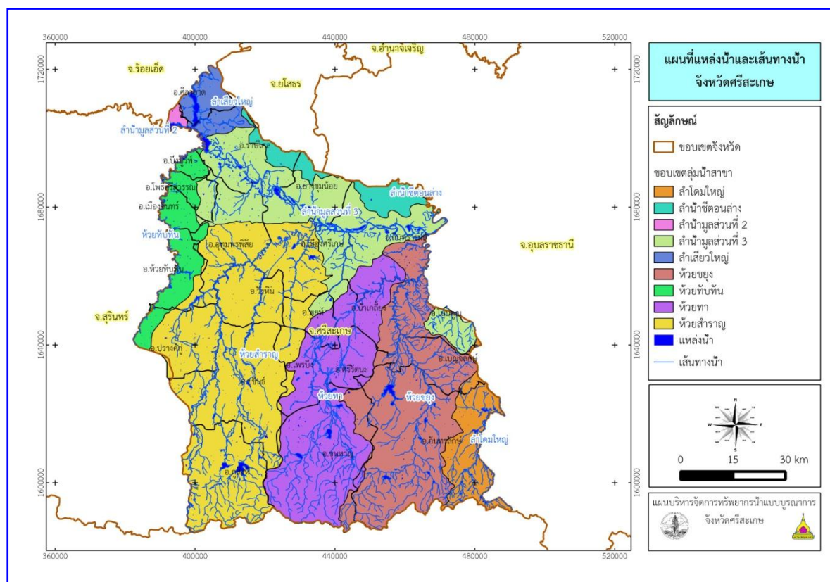
แผนภาพที่ ๑๓ แผนที่เส้นทางน้ำ แหล่งน้ำ และขอบเขตลุ่มน้ำสาขาในพื้นที่จังหวัดศรีสะเกษ
