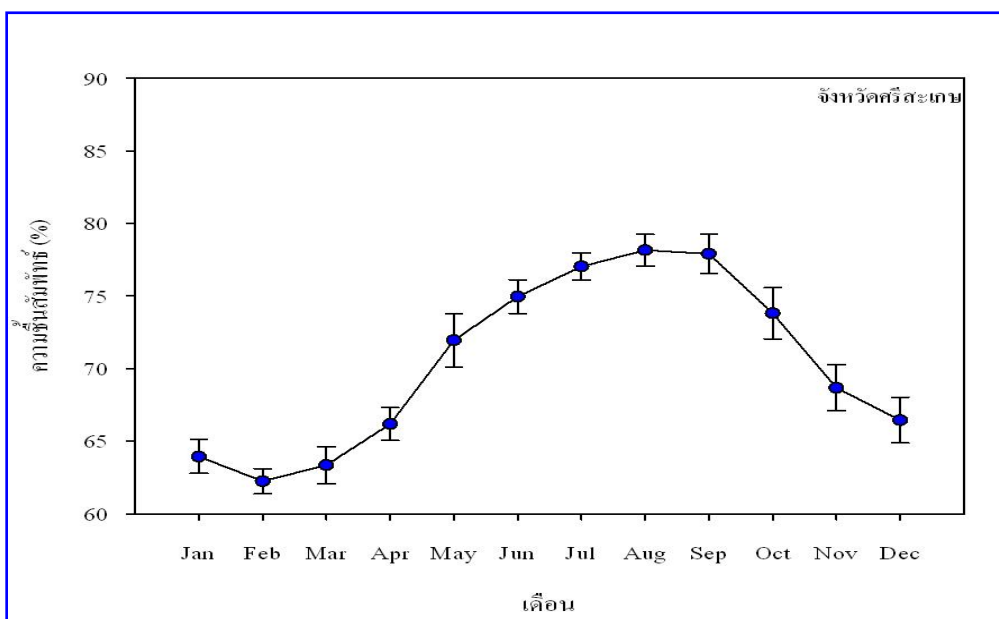
แผนภาพที่ ๓ กราฟแสดงค่าร้อยละของความชื้นสัมพัทธ์ (ค่าเฉลี่ย ๑๐ ปี ระหว่าง พ.ศ. ๒๕๔๒-๒๕๕๑) ที่มา : กรมอุตุนิยมวิทยา อ้างถึงโดยศูนย์วิจัยข้าวสุรินทร์ (๒๕๕๗)
