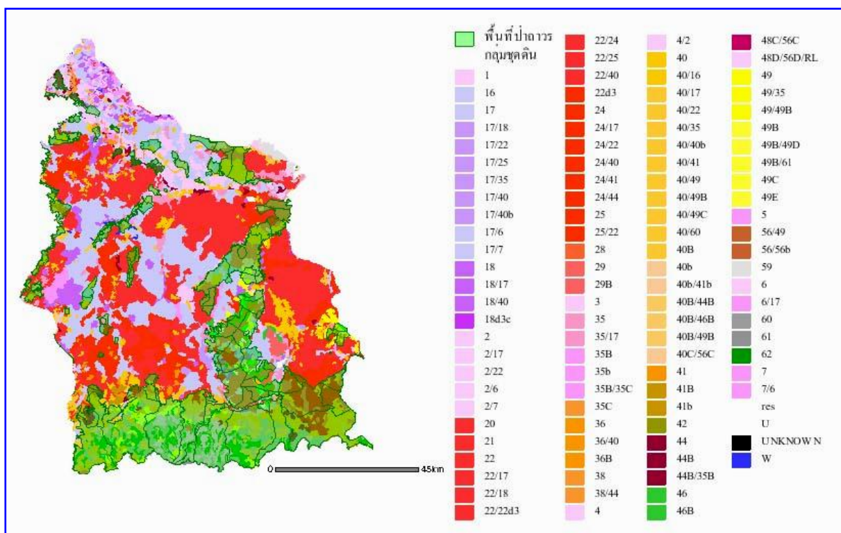
แผนภาพที่ ๙ แผนที่กลุ่มชุดดินของจังหวัดศรีสะเกษ
