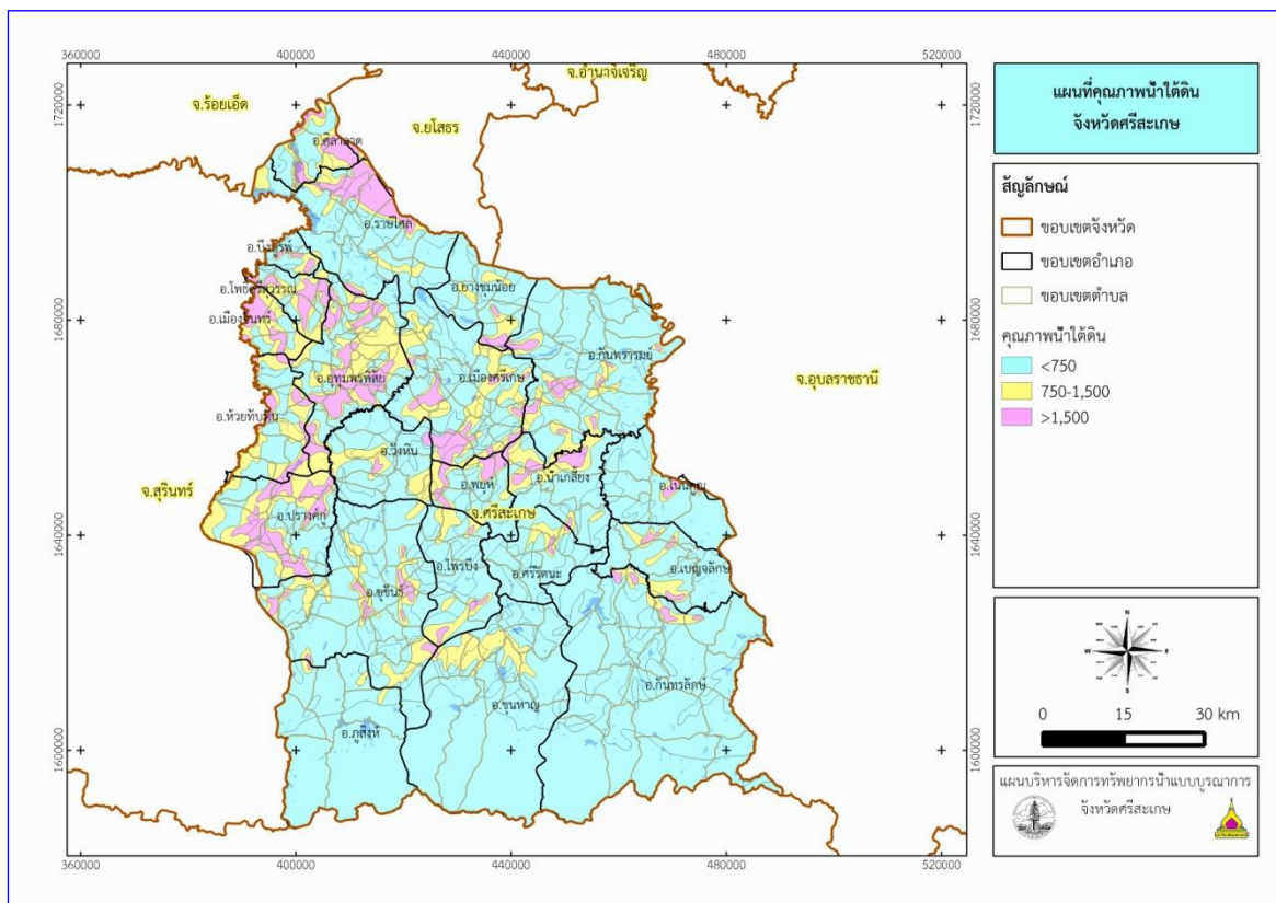
แผนภาพที่ ๑๕ แผนที่แสดงคุณภาพน้ำใต้ดินของจังหวัดศรีสะเกษ
