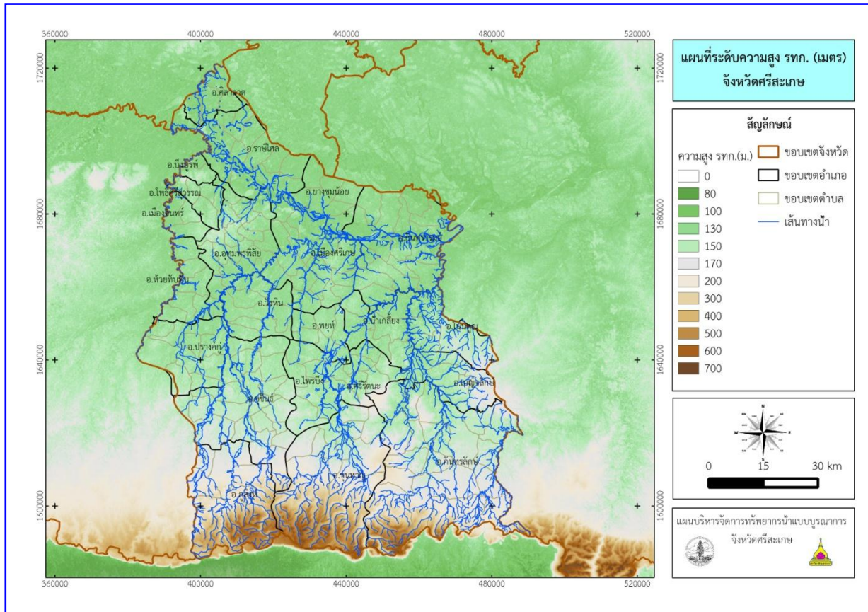
แผนภาพที่ ๑ แผนที่สภาพภูมิประเทศด้านระดับความสูงของพื้นที่จังหวัดศรีสะเกษ
