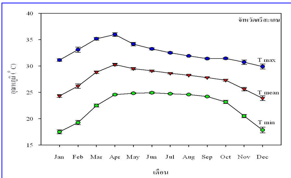
แผนภาพที่ ๒ กราฟแสดงอุณหภูมิเฉลี่ยในแต่ละเดือนของจังหวัดศรีสะเกษ ประกอบด้วย อุณหภูมิสูงสุด (T_max) ต่ำสุด (T_min) เฉลี่ย (T_mean) (ค่าเฉลี่ย ๑๐ ปี ระหว่าง พ.ศ. ๒๕๔๒-๒๕๕๑) ที่มา : กรมอุตุนิยมวิทยา อ้างถึงโดยศูนย์วิจัยข้าวสุรินทร์ (๒๕๕๗)
